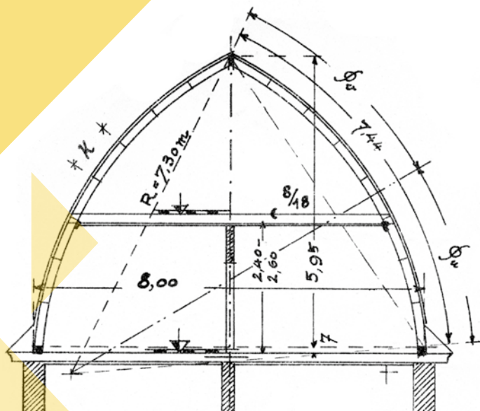
Zollinger-Dachkonstruktion
